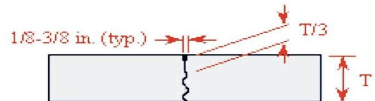
Untied - Longitudinal (Type A-3)
